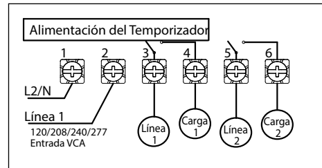
ET1725 configurado para cargas DPST con cable puente ajustado en SIM
