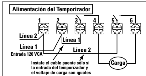
ET1725 configurado para carga DPST 240 V CA con cable puente ajustado en SIM
