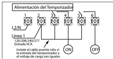
ET1725 configurado para carga SPST de pulso con cable puente ajustado en PUL
