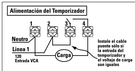
ET1705 configurado para SPST, carga de 120 V CA
