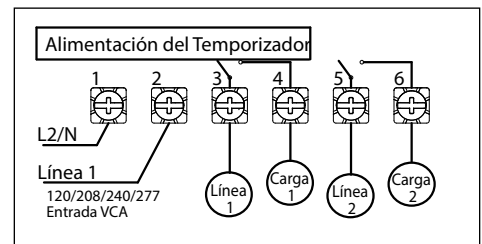
ET1725 configurado para 2 cargas SPST con cable puente ajustado en IND
